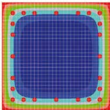
Andamento della temperatura in un pilastro in cemento armato
